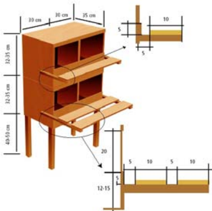
Рис. 1: размеры гнезда
